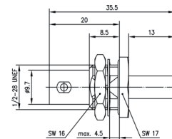
BNC-Stecker <> BNC-Einbaubuchse
